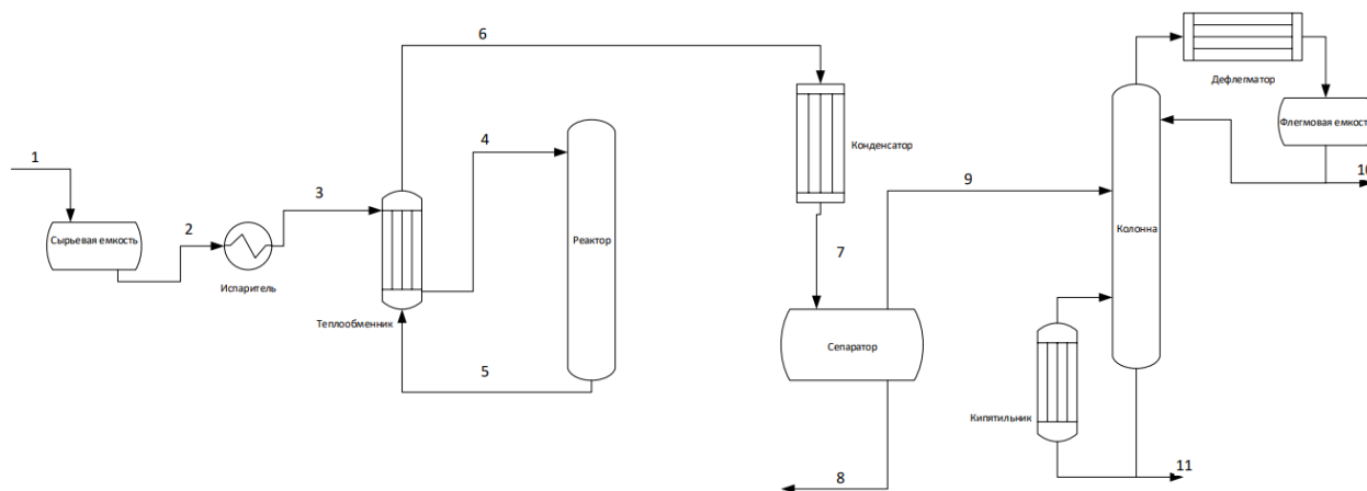
Рисунок 1 – Принципиальная технологическая схема химико-технологического процесса
